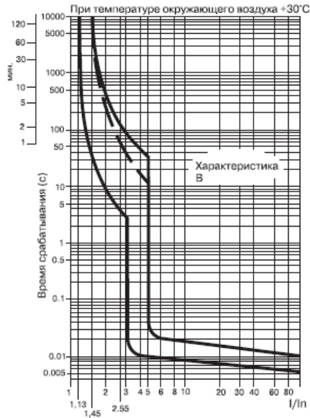
Рисунок 1 — Времятоковые характеристики срабатывания ВА47-29 от сверхтока.
