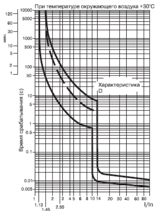
Рисунок 3 — Времятоковые характеристики срабатывания ВА47-29 от сверхтока.
