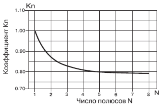
Рисунок 5 — Зависимость коэффициента K_n от числа полюсов
