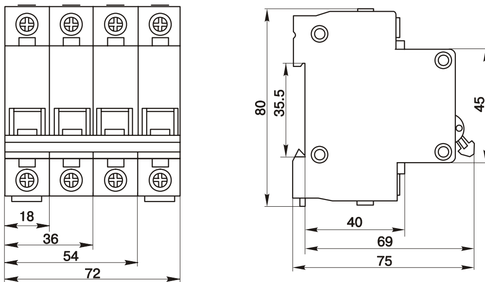
Рисунок 6 — Габаритные и установочные размеры ВА47-29
