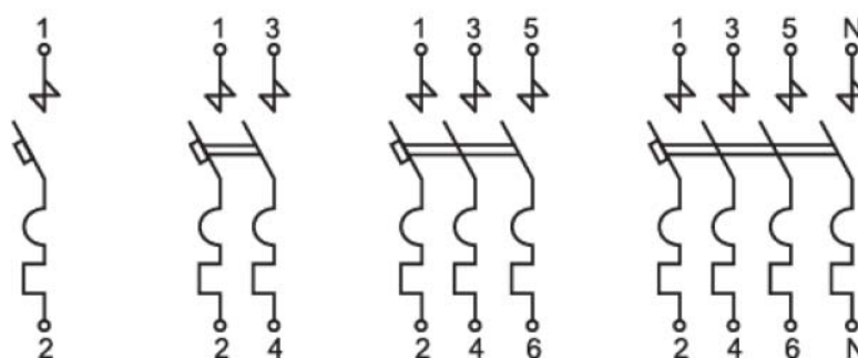
Рисунок 7 — Электрические схемы ВА47-29
