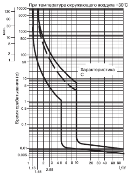
Рисунок 2 — Времятоковые характеристики срабатывания ВА47-29 от сверхтока.
